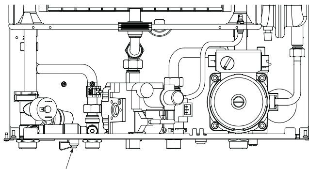
Válvula de enchimento do circuito
